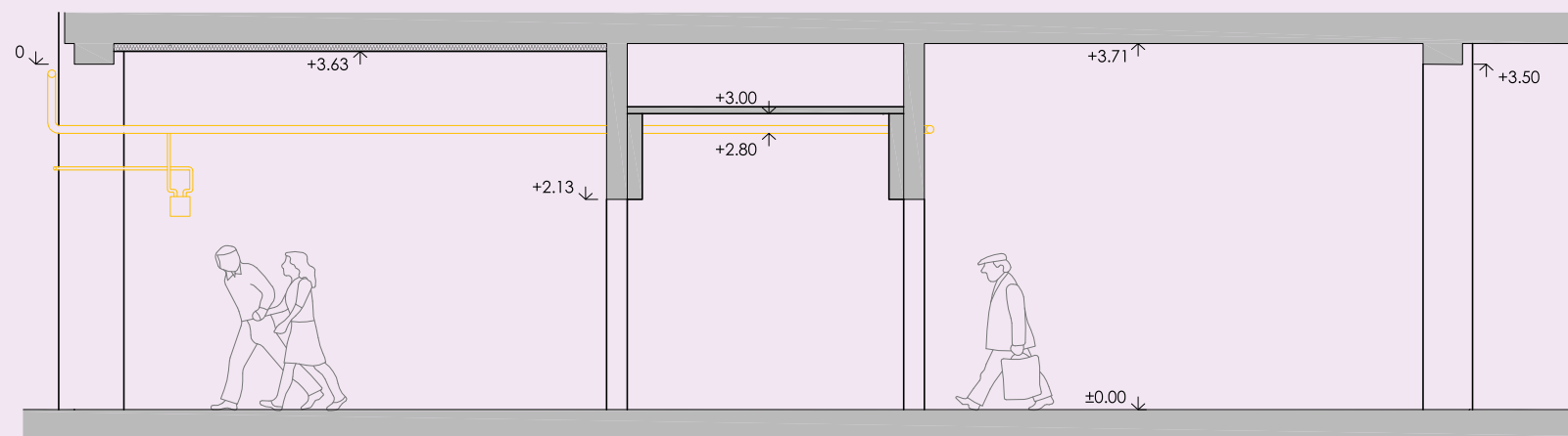
S01 - S01
