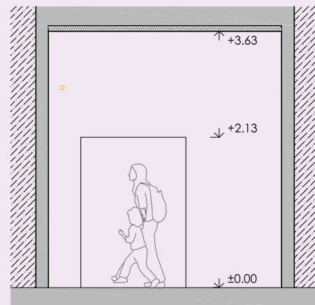
S04 - S04
